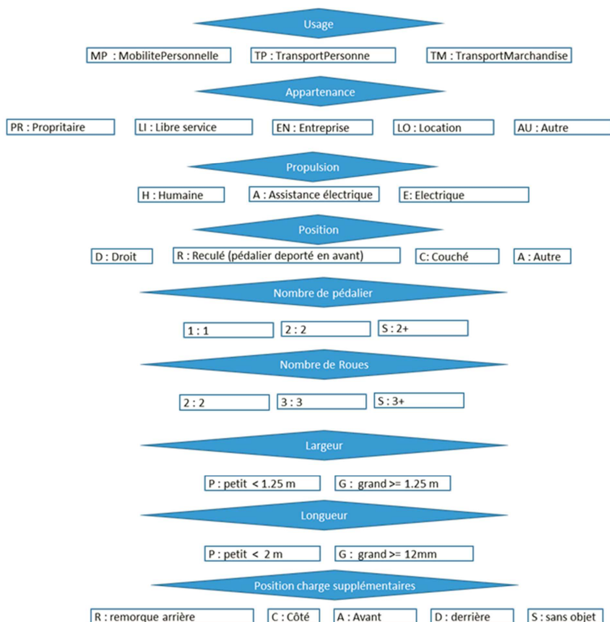
Figure 4.5.2 : Dimensions de codage des vélos
