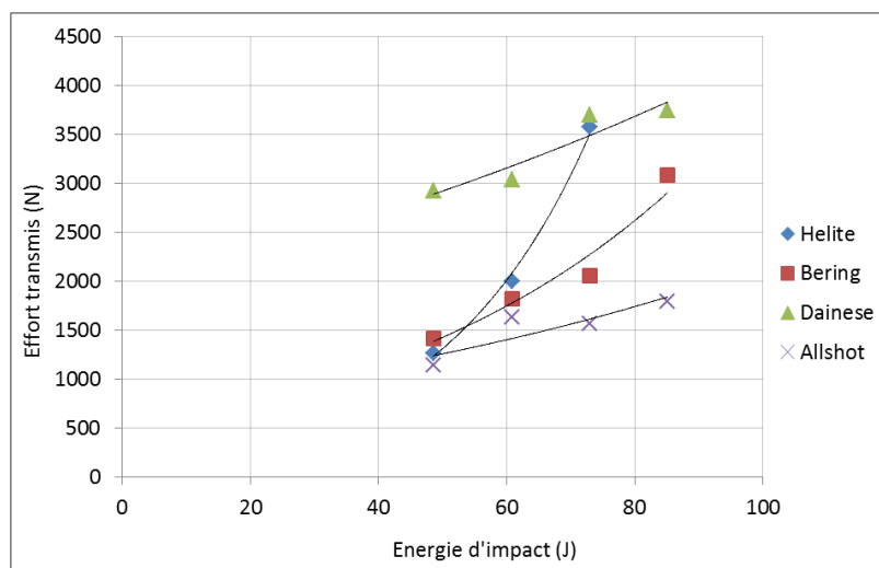
Figure 15 : Effort transmis au travers de gilets airbag en fonction de l'énergie d'impact
