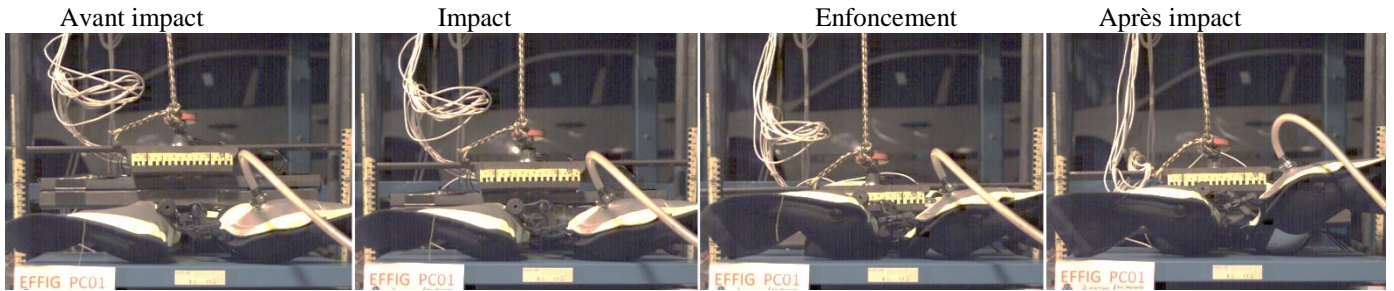
Figure 14 : Impact avec une énergie de 50J sur un gilet Helite gonflé à 0,3 bar
