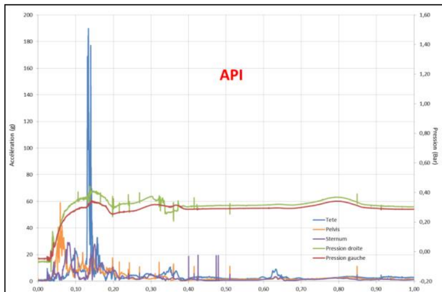
Figure 24 : Courbes des pressions de l'airbag « API » au cours du crash-test et accélérations subies par le sujet
