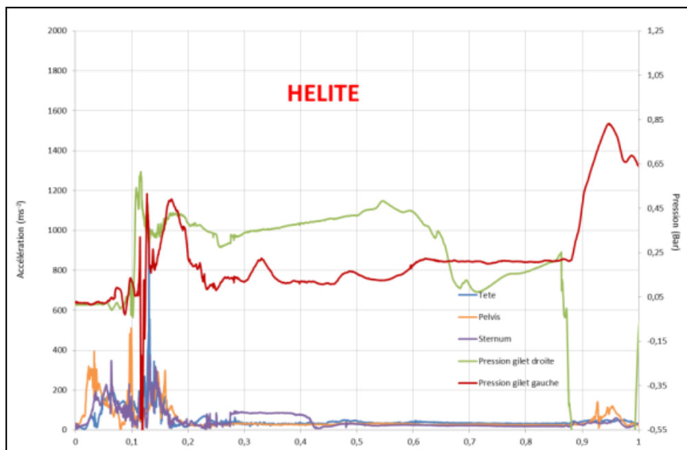
Figure 20 : Courbes des pressions de l'airbag « Helite » au cours du crash-test et accélérations subies par le sujet
