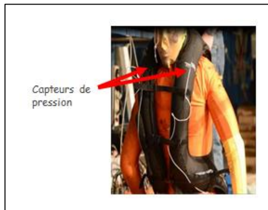
Figure 12 : Essai de gonflage du gilet airbag « Helite »
