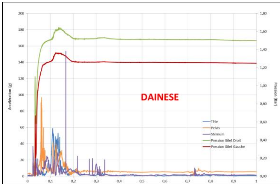
Figure 23 : Courbes des pressions de l'airbag « Dainese » au cours du crash-test et accélérations subies par le sujet
