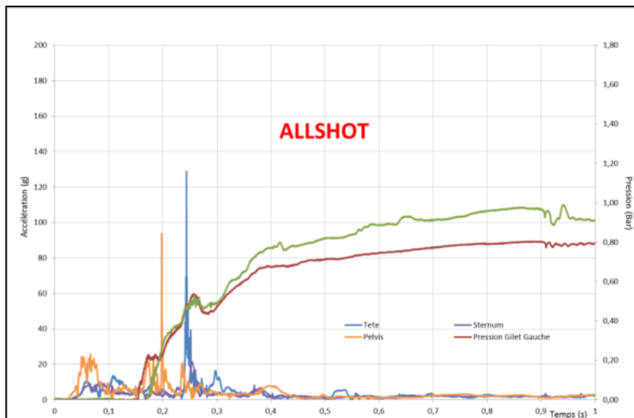
Figure 19 : Courbes des pressions de l'airbag « Allshot » au cours du crash-test et accélérations subies par le sujet
