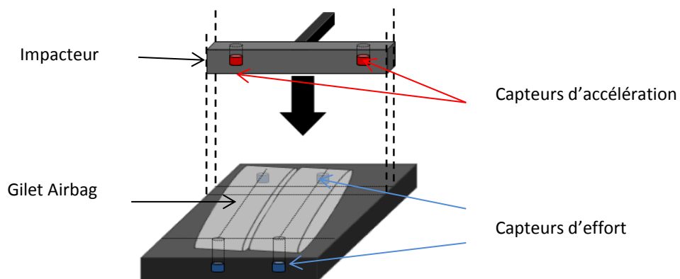
Figure 13 : montage expérimental
